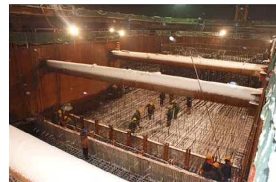
主墩承台施工现场
